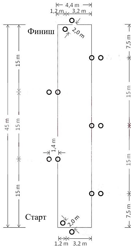
Рисунок 108. Схема этапа «слалом»
