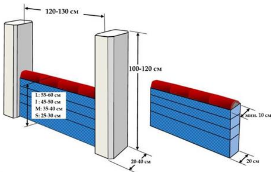
Рисунок 126. Конструкция препятствия «стенка»
