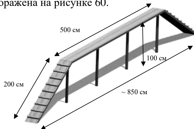
Рисунок 60. Схема препятствия «бум»
