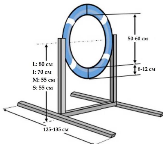
Рисунок 132. Конструкция препятствия «шина»
