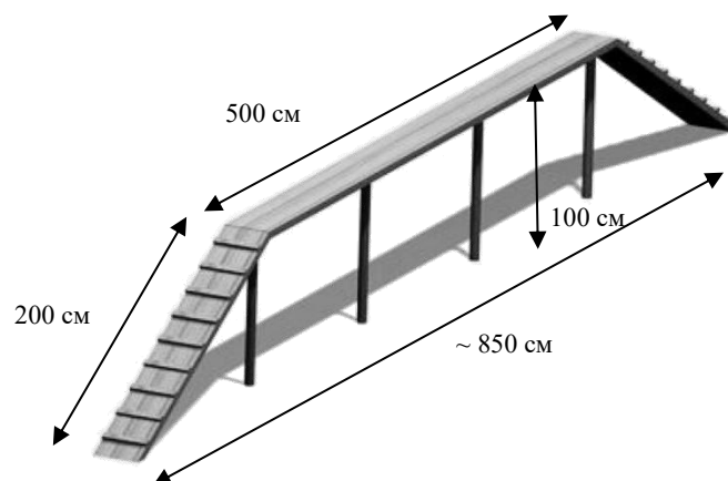
Рисунок 34. Схема препятствия «бум»
