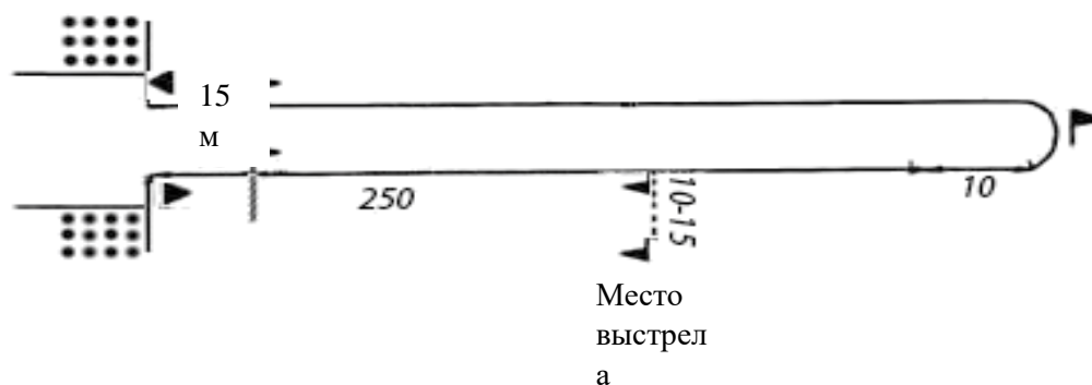
Рисунок 88. Трасса буксировки на открытой местности
