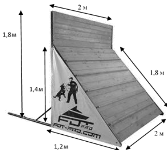
Рисунок 57. Схема препятствия «глухой забор»
