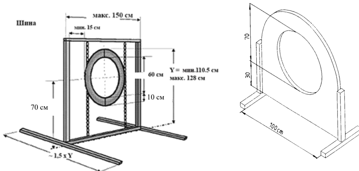
Рисунок 101. Шина
