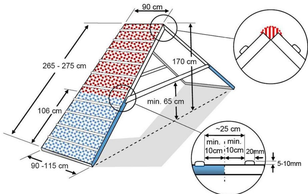
Рисунок 129. Конструкция препятствия «горка»
