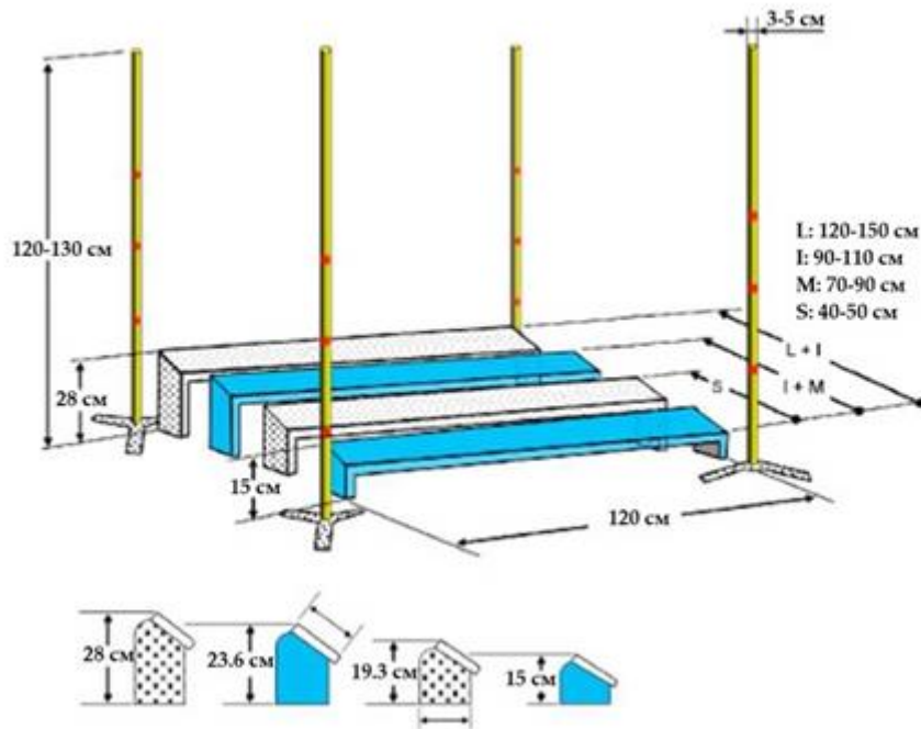
Рисунок 133. Конструкция препятствия «прыжок в длину»
