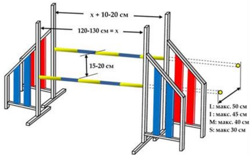
Рисунок 125. Конструкция препятствия «двойной барьер»
